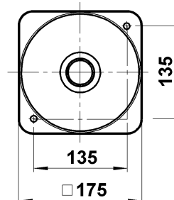
Bohrbild für Leuchtenfuß
